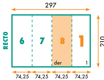
Pli économique (2 plis / 4 volets)
